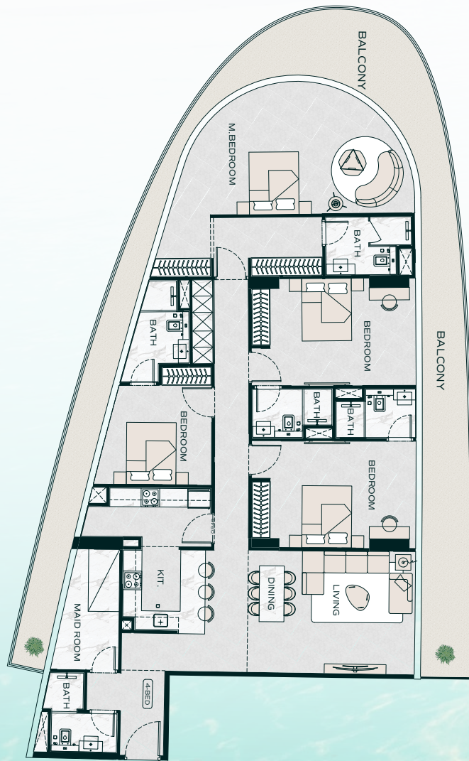
4 BEDROOM TYPE 01
