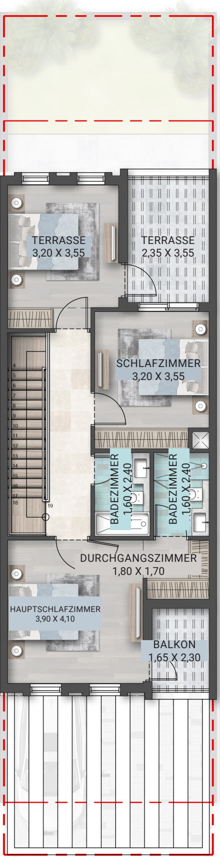
1. OBERGESCHOSS
