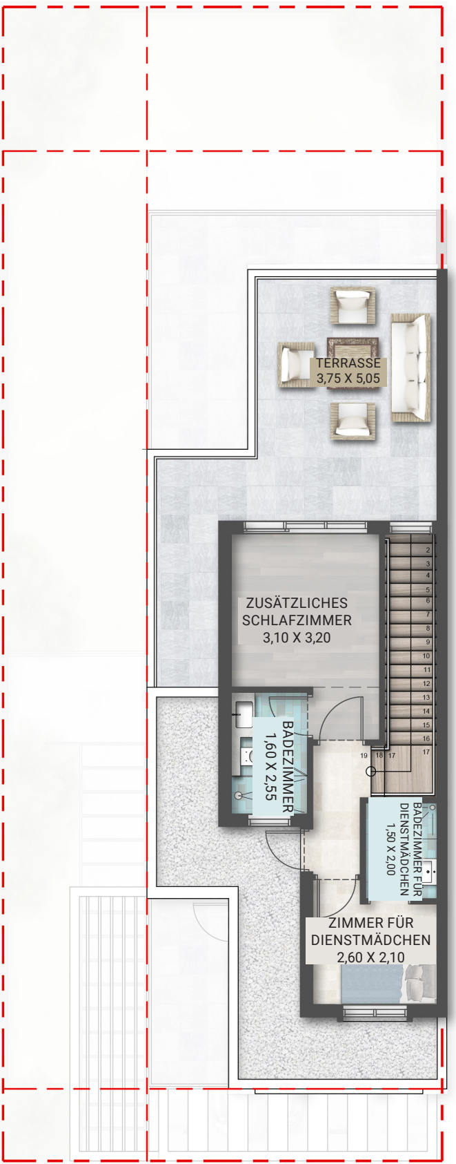
2. OBERGESCHOSS
