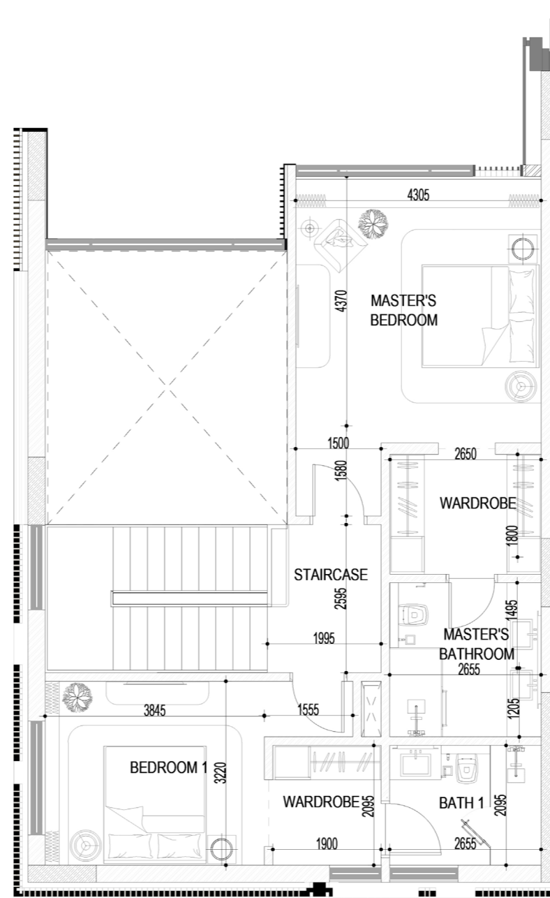
3 BED - DUPLEX 401
