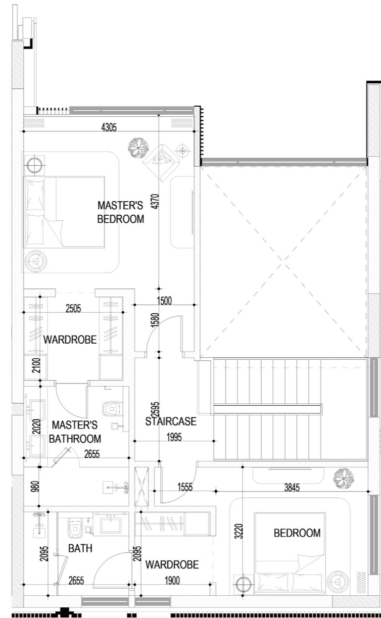
3 BED - DUPLEX 306
