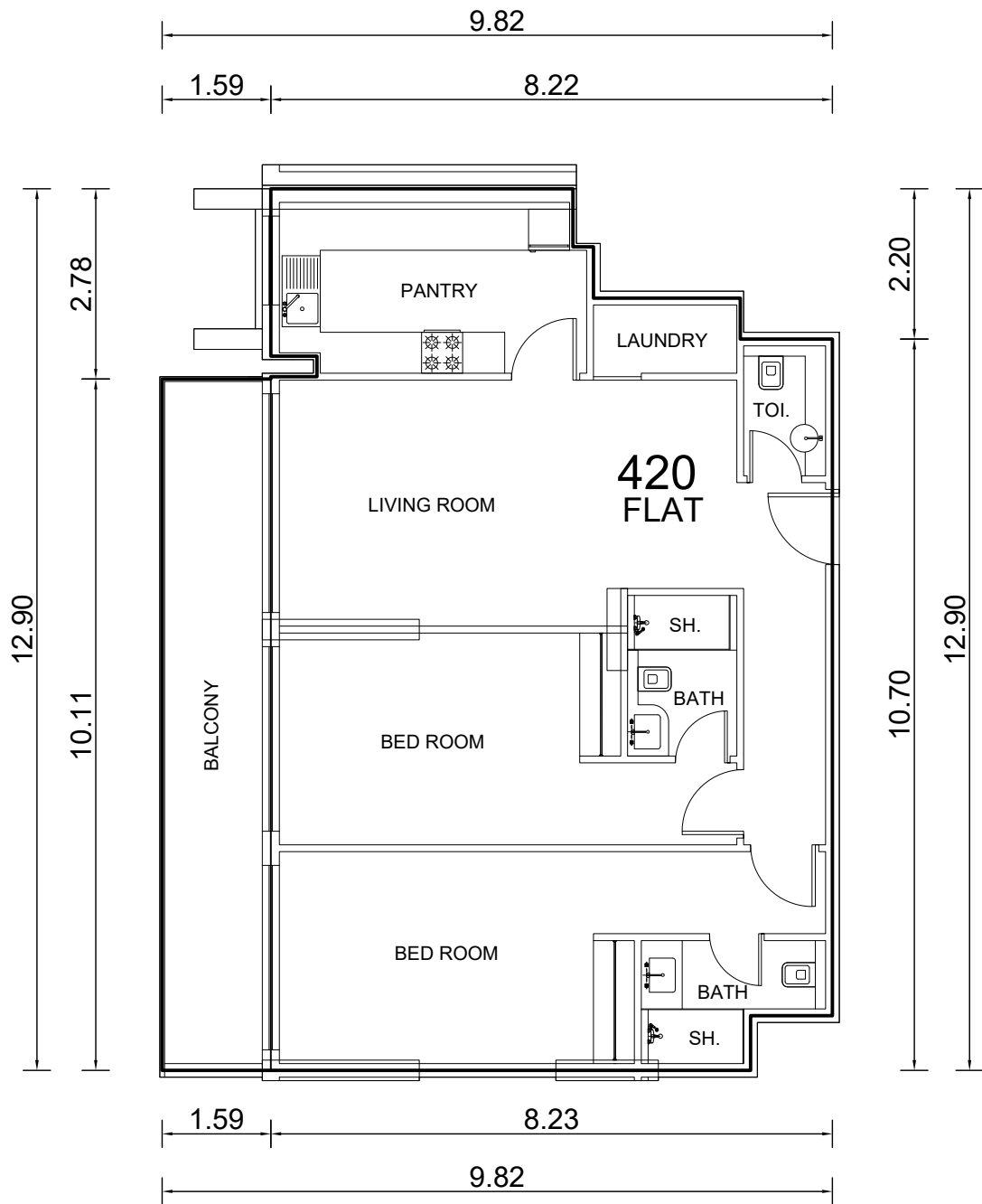
UNIT DETAIL SCALE: 1:100
