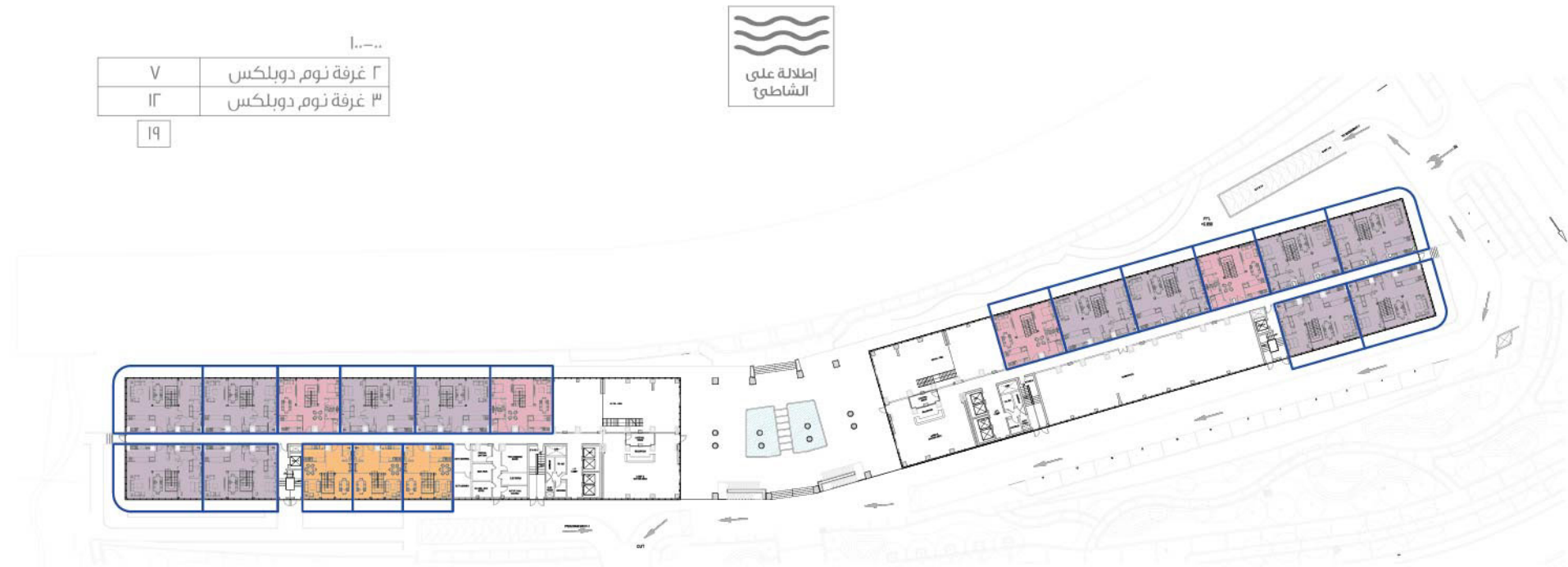
الطابق الأرضي
